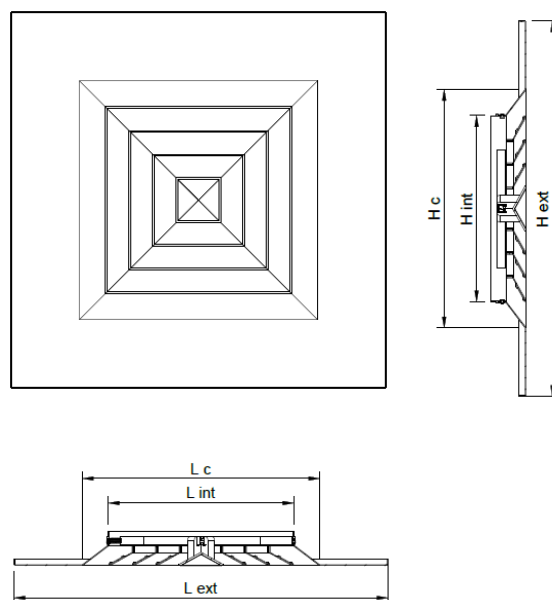
Anemostat ramă lată
